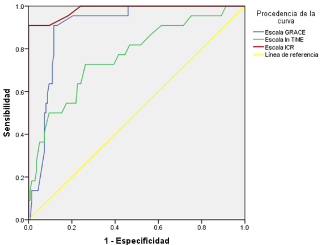
GRÁFICO 1. Curvas ROC de las escalas GRACE, In Time e ICR
