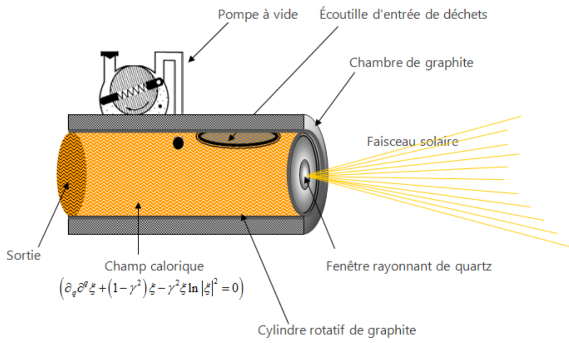
Fig. 14: Représentation schématique de la chambre de pyrolyse du réacteur solaire.
