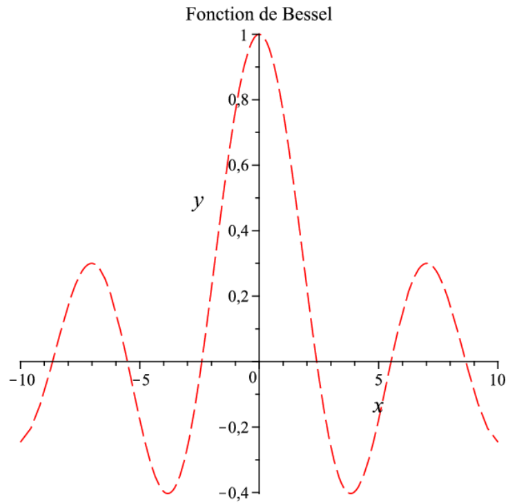
Fig. 5: Solution pour l'équation de Lane-Emden cylindrique.
