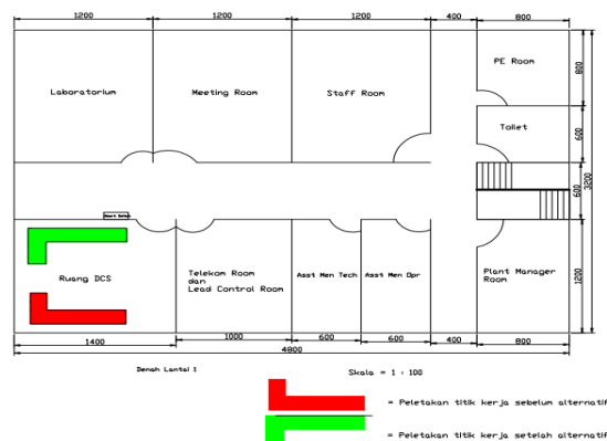
Gambar 1 Peletakkan Lantai 1
