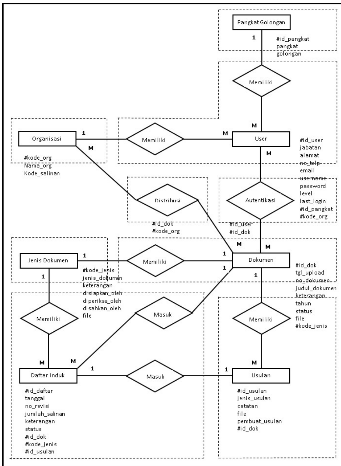
Gambar 6. Transformasi ERD ke LRS
