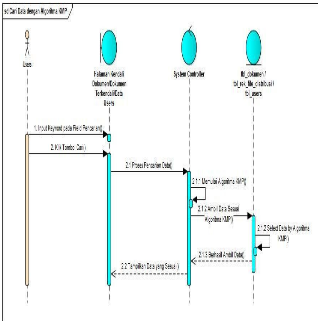
Gambar 21. Sequence Diagram Cari Data dengan Algoritma
