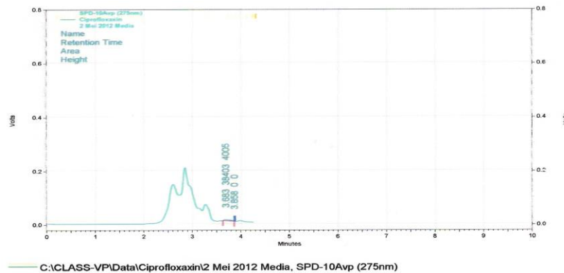
Gambar 2. Profil kromatogram media MHB, menggunakan kolom C18 dengan suhu kolom 42°C, panjang gelombang 275 nm, dan fase gerak buffer natrium dihidrogen fosfat pH 3,0 : asetonitril (65:35, v/v)
