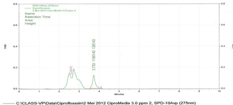
Gambar 3. Profil kromatogram siprofloksasin 3,0 µg/mL dalam media MHB, menggunakan kolom C18 dengan suhu kolom 42°C, panjang gelombang 275 nm, dan fase gerak buffer natrium dihidrogen fosfat pH 3,0 : asetonitril (65:3, v/v)
