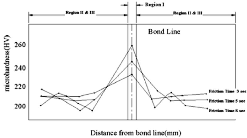
Gambar 2 pengujian kekerasan AISI 304 (Sathiya dkk, 2004)
