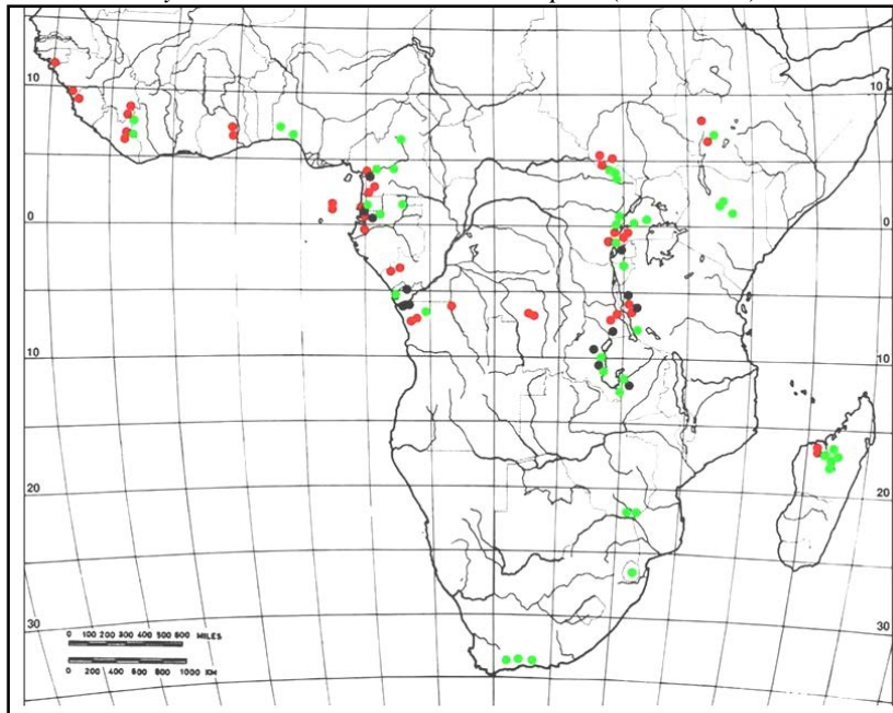
Figure 3. Exemple des trois espèces de liaison des régions afromontagnarde/afro-tropicale : Amauropelta oppositifomis (ronds verts), Antrophyum mannianum (ronds rouges) et Cyathea camerooniana var. aethiopica (ronds noirs).
