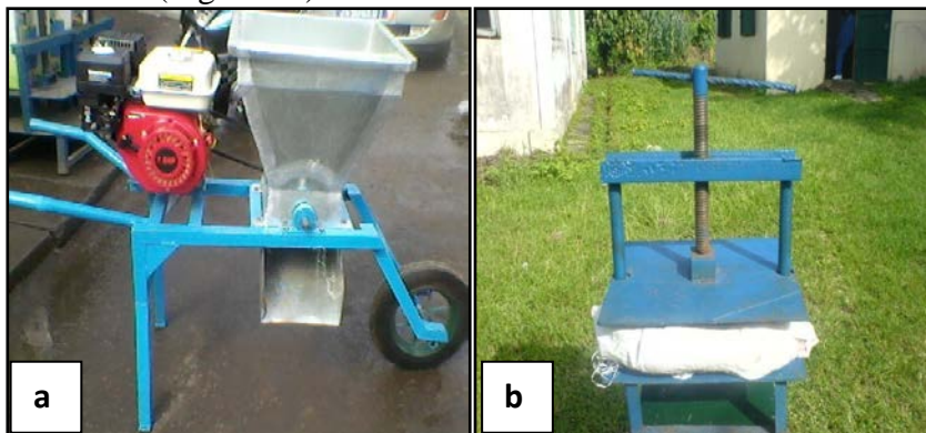
Figure 1: Matériel de broyage et de pressage du manioc. a : Broyeur ; b : Presse à vis.
