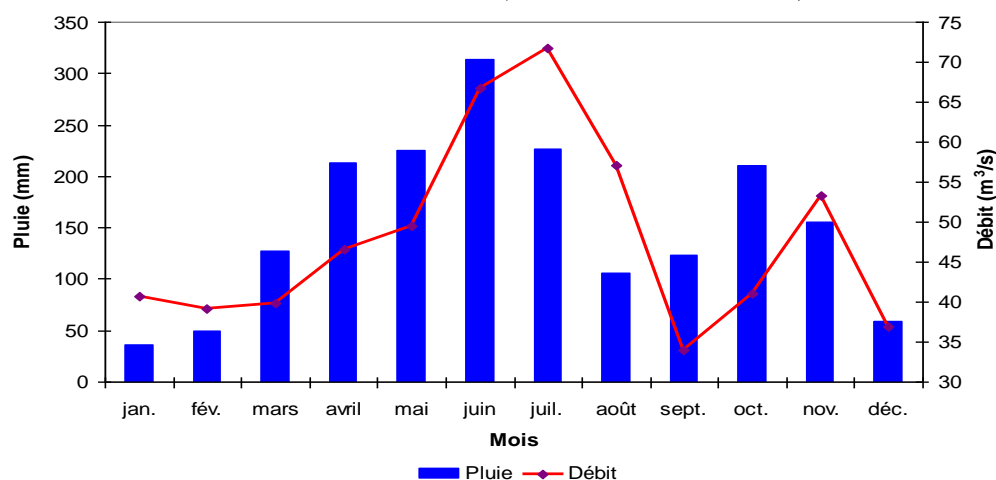
Figure 2. Variations des moyennes mensuelles de la pluie et des débits de la rivière Bia de 1990 à 2007 (Sources : Société d'exploitation de développement aéroportuaire, aéronautique et météorologique (SODEXAM) et Direction Générale des Infrastructures de l'Hydraulique Humaine (DGIHH))
