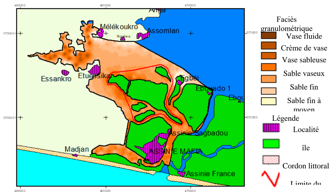
Figure 7. Répartition des faciès de surface des sédiments de la lagune dans la zone du Parc national des îles Ehotilé
