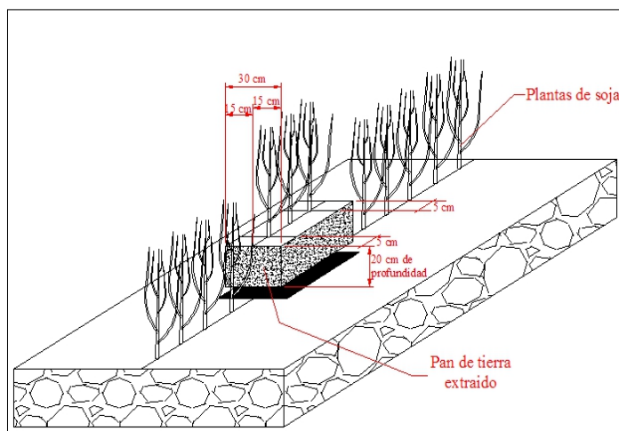
Figura 1. Diagrama de la extracción del pan de tierra para la determinación de crecimiento de raíces y nodulación de plantas de soja.
