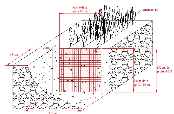
Figura 2. Diagrama de ubicación de la grilla metálica en la calicata para el cartografiado y determinación de DLR en raíces de soja
