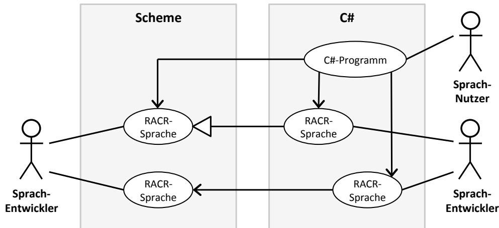
Abbildung 3.1.: Anwendungsfälle von RACR in Scheme und C#
