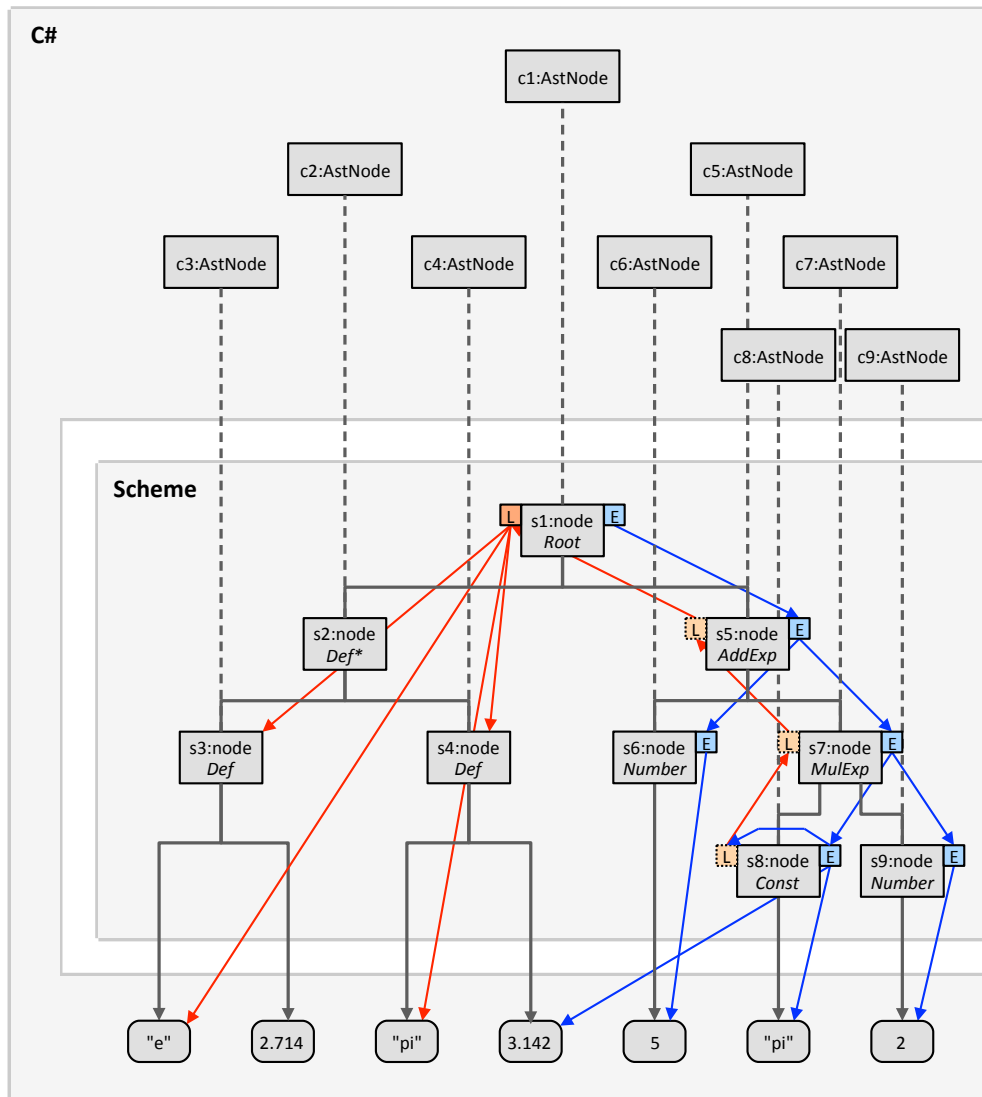
Abbildung 4.1.: Beziehungen zwischen Adapter-Objekten und node -Records im AST
