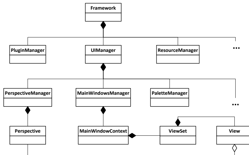
Рис. 3. Основные компоненты ядра VTMine
