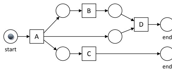
Рис. 2. Модель сети Петри для исполнения схемы на рис. 1б
