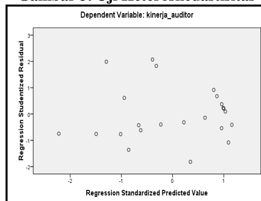
Gambar 3. Uji Heteroskedastisitas
