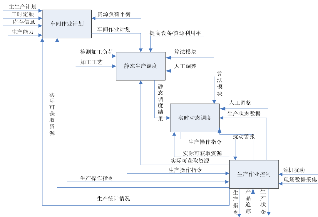
圖 2 生產作業計畫和調度控制的流程圖
