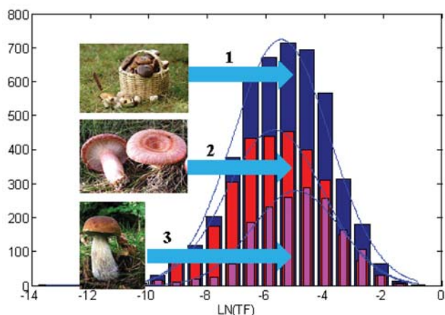
Рис. 6. Частотные распределения логарифмов коэффициентов перехода ^{137}\text{Cs} в грибы разных видов по данным НИИРГ и по своим собственным данным за период с 1987 по 2009 г.: 1 – грибы с пластинчатым и трубчатым гименофором; 2 – грибы с пластинчатым гименофором; 3 – грибы с трубчатым гименофором
