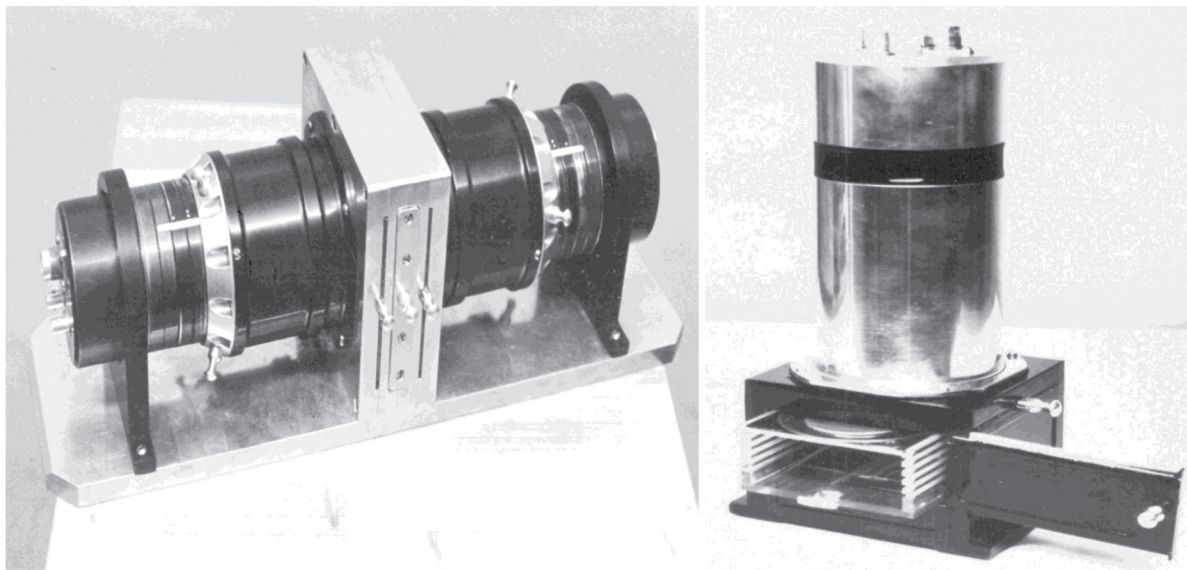
Рис. 1. Детекторы альфа-излучения (слева – для двухсторонней радиометрии)
