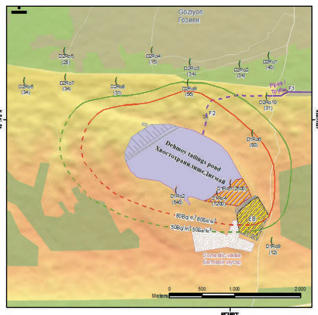
Рис. 1. ОА радона в воздухе на хвостохранилище Дигмай и вокруг него
