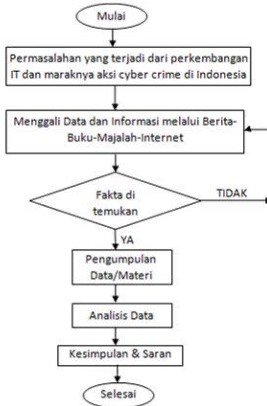
Gambar 1. Kerangka Pemikiran
