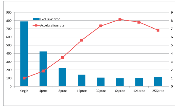
図 7 並列化性能
