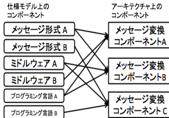
図1 仕様モデルのコンポーネントとアーキテクチャのコンポーネントの関係
