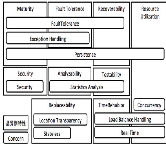
図8 ISO9126の品質特性と特定した関心事(一部)
