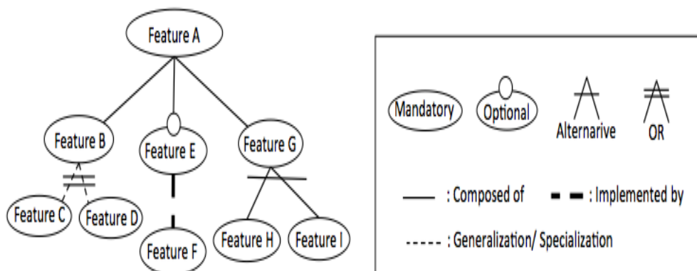
図5 フィーチャ図の構成
