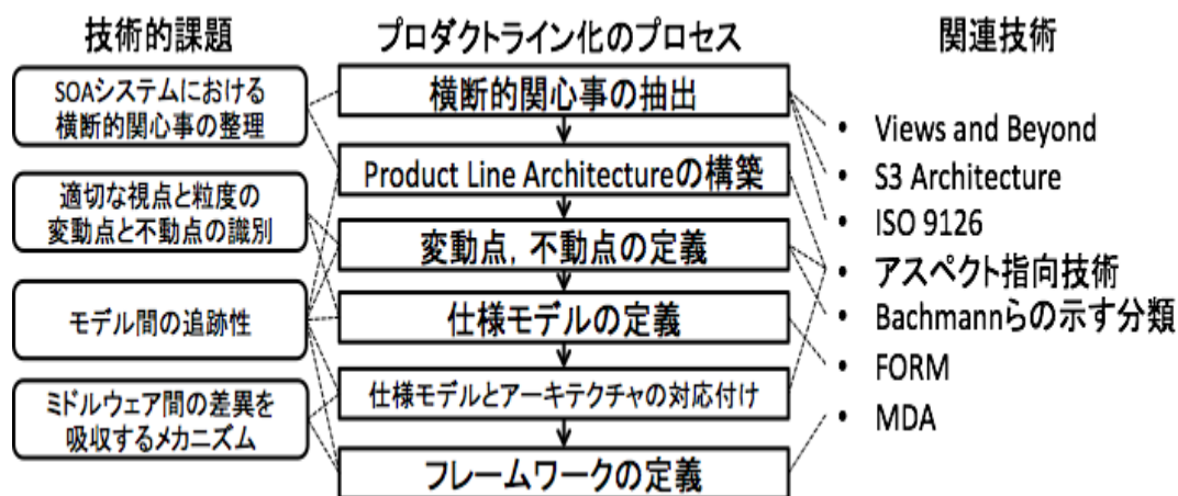
図2 プロダクトライン化の手順と関連技術
