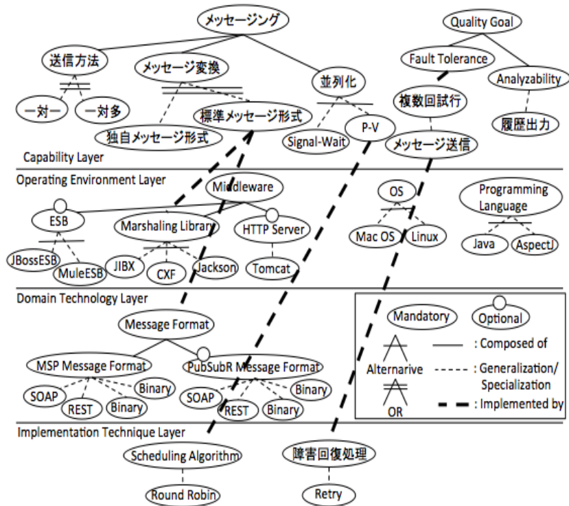
図 11 アプリケーションプラットフォームの仕様モデル (一部)
