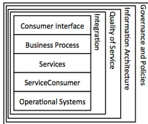
図4 S3 Architecture の階層構造
