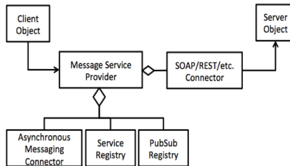
図3 SOA スタイルを基本構造としたアプリケーションプラットフォームの構造
