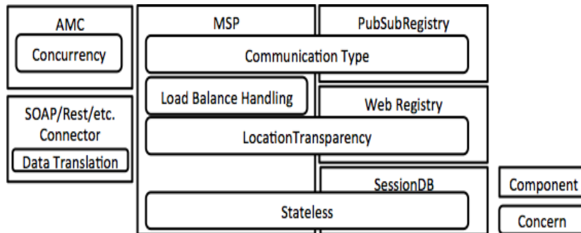
図6 SOA スタイルの構造と特定した関心事 (一部)
