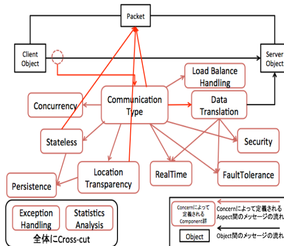
図9 アプリケーションプラットフォームのプロダクトラインアーキテクチャ
