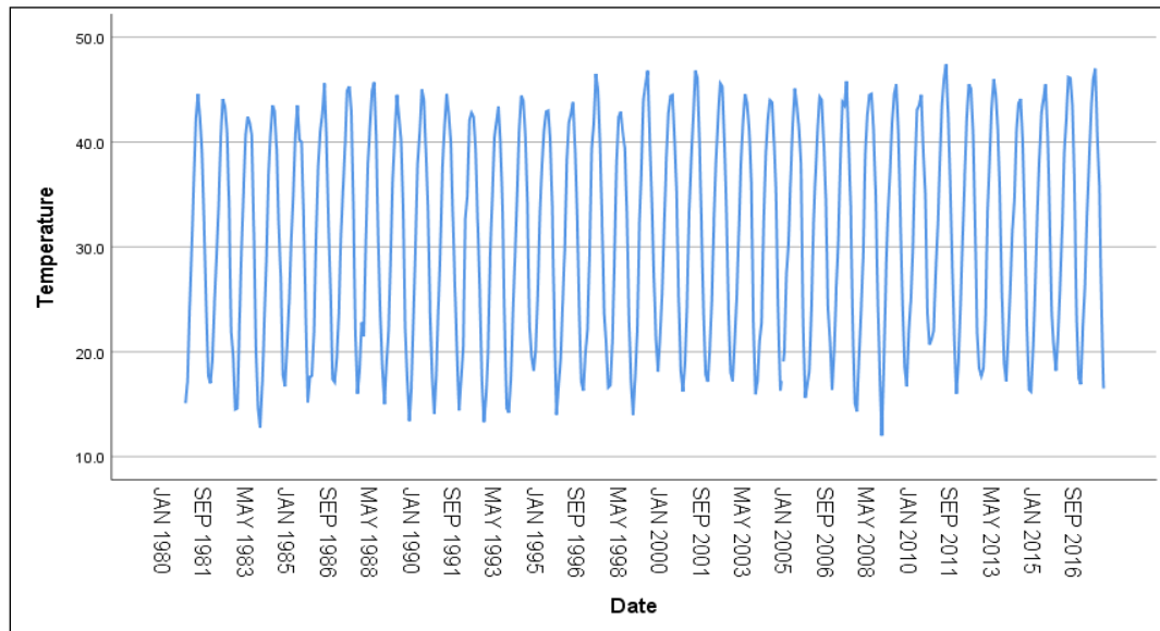
Fig.2: Monthly Max. Temperature of Kerbala (Jan.1980 - Dec.2016)
