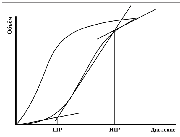
Рис. 1. Схематическое изображение точки нижнего перегиба на кривой объем-давление.
