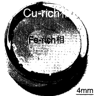
図2 Cu-26Fe-4V (wt.%)合金のインゴットの外観写真
