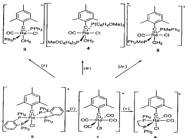
Scheme 1 - (i) pdpp; (ii) PPh 3 ; (iii) P(C 6 H 4 OMe) 3 ; (iv) PMePh 2 ; (v) dppe.
