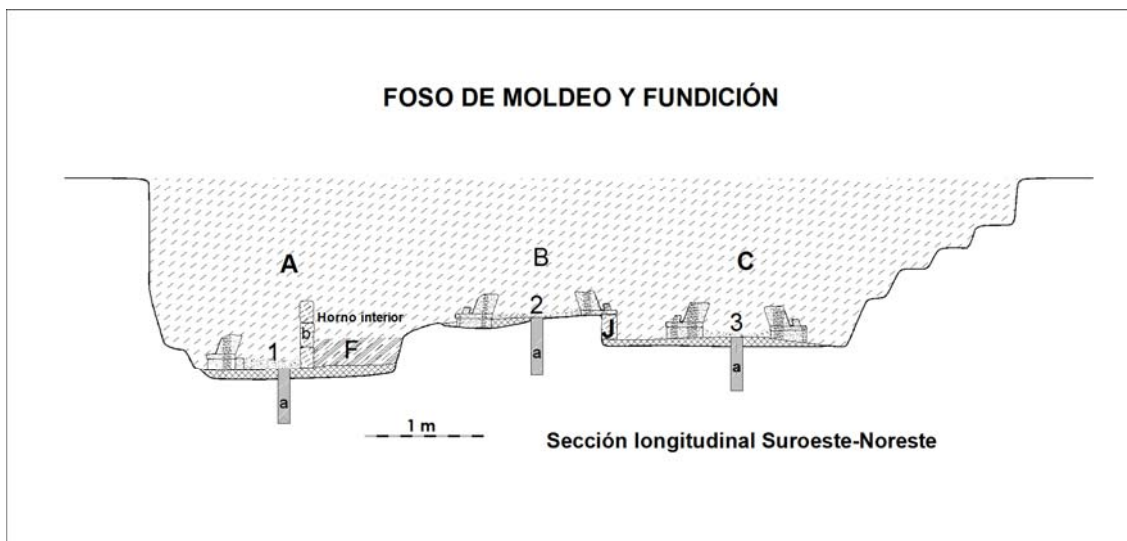
Fig. 3: Sección longitudinal del foso de moldeo y fundición
