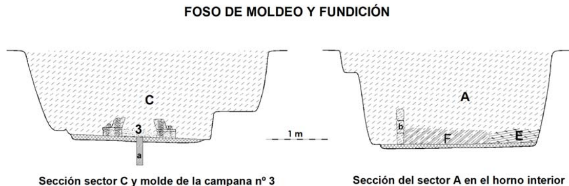
Fig. 4: Secciones transversales del foso de moldeo y fundición
