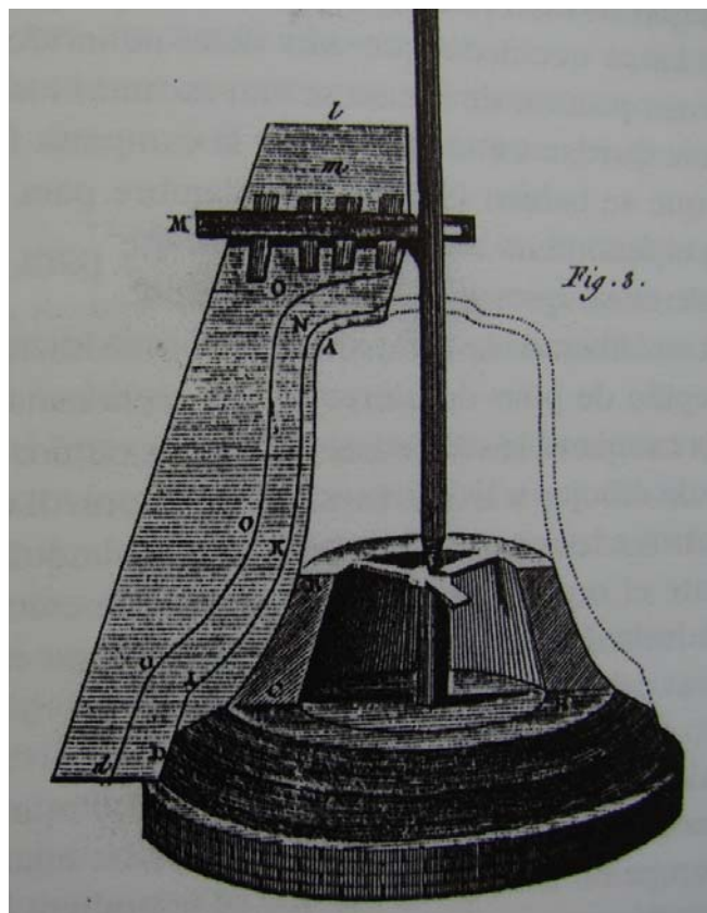
Fig. 7: Terraaja y sección de los moldes de una campana. Ilustración de la Enciclopedia de Diderot y D'Alambert
