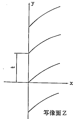
図2 直線翼列
