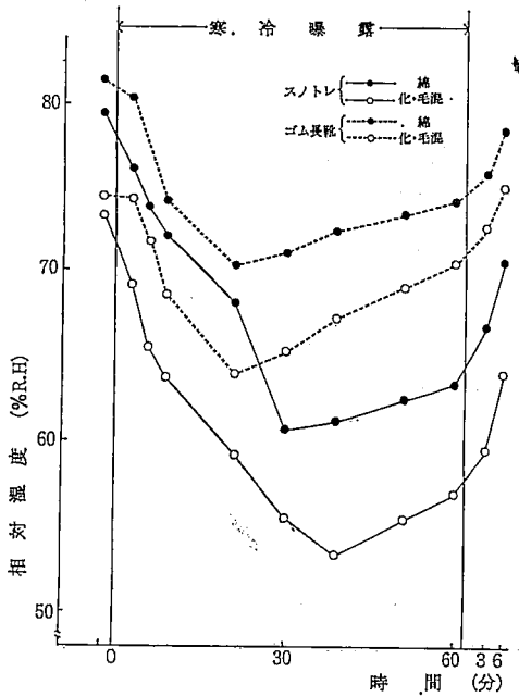
図6 ソックス内相対湿度の経時変化
