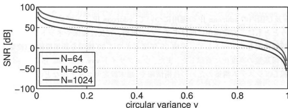
位相スペクトル差の円周分散 (circular variance) に対する POC 関数の SNR ( N : 信号長)
