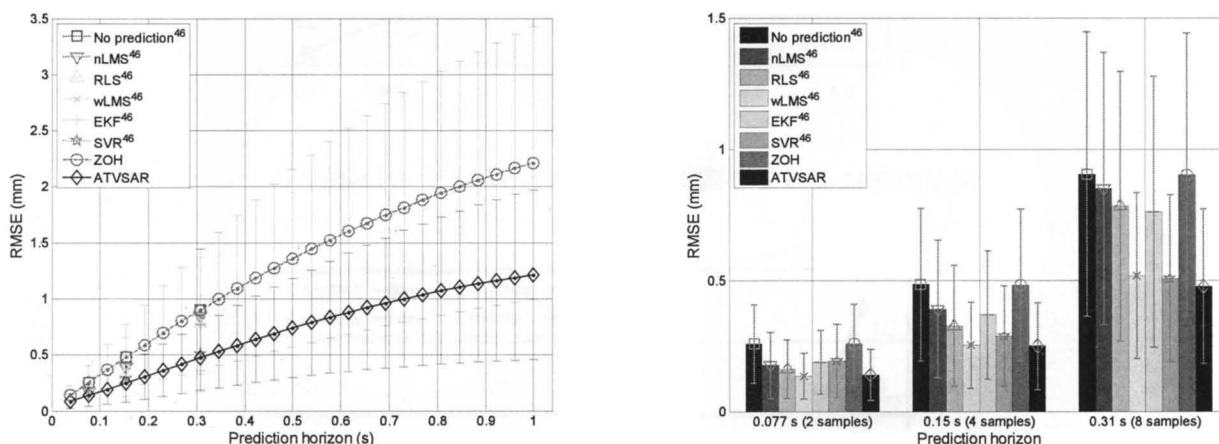
(左) 304 例の加工済みデータセットにおける平均予測誤差と、(右) ATVSAR と最新の予測法複数との比較 (左図より 77 ms, 150 ms, 310 ms を抜粋)
