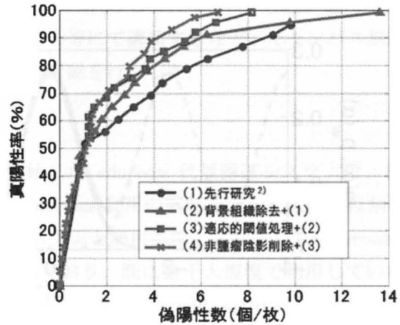
FROC 曲線による性能比較結果
