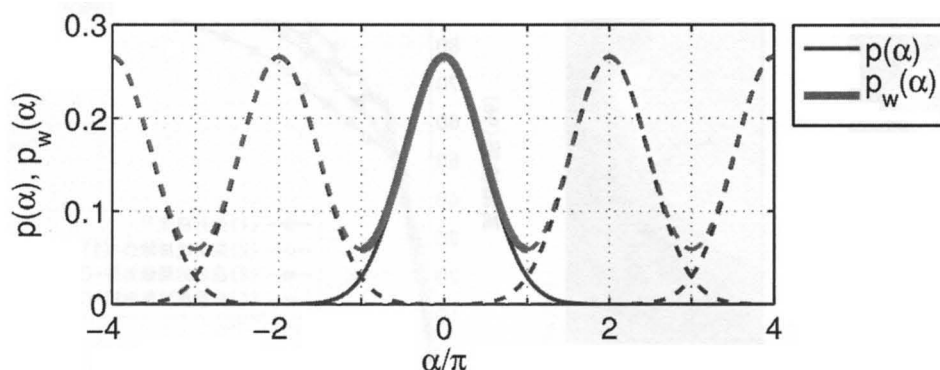
線形確率分布の確率密度関数 p(\alpha) と巻き込み分布の確率密度関数 p_w(\alpha)
