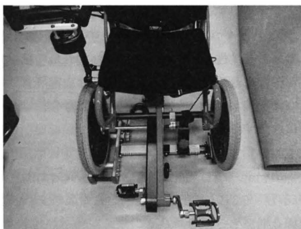
新しいバーチャルリアリティシステムの筐体（足こぎ車いす搭載時）
