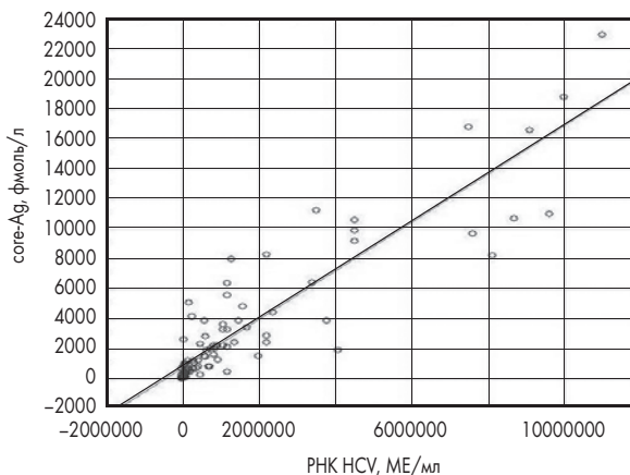
Рисунок 1. Корреляционная зависимость между концентрациями core-Ag и вирусной РНК
