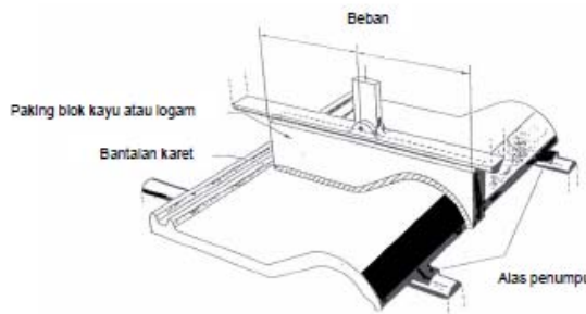
Gambar 2 Cara Uji Beban Lentur untuk Genteng Profil
