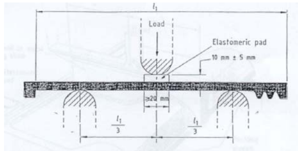
Gambar 1 Cara Uji Beban Lentur untuk Genteng Rata
