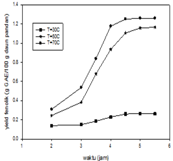
Gambar 8. Hubungan Antara Waktu Terhadap Yield Phenolic Pada Berbagai Suhu Ekstraksi
