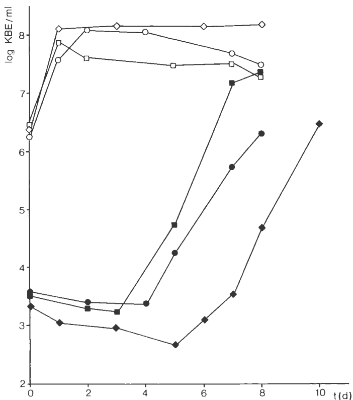
Abb. 5: Killertoxinwirkung von Hanseniaspora uvarum 470 auf Saccharomyces cerevisiae 381 in Mischkultur bei verschiedenen Temperaturen. Koloniebildende Einheiten (KBE/ml) von H. uvarum (konturierte Symbole) und S. cerevisiae (ausgefüllte Symbole); B-Medium, pH 3,5. — ◇/◆ 20 °C, ○/● 25 °C, □/■ 30 °C.
