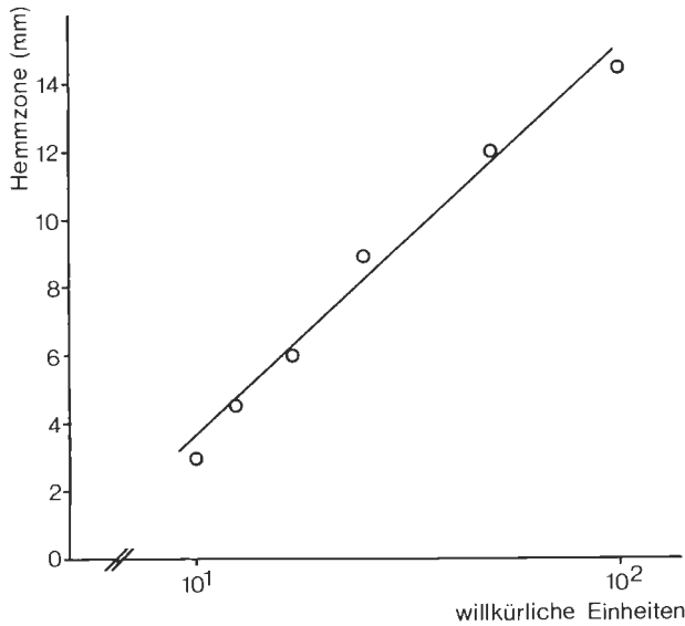
Abb. 1: Eichdiagramm für die Killertoxinaktivität von Hanseniaspora uvarum 470. Calibration curve for the activity of the killer toxin of H. uvarum 470.
