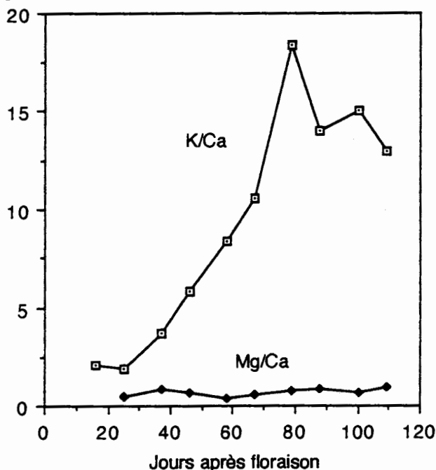
Fig. 1: Evolution des rapports K/Ca et Mg/Ca dans la baie entière au cours du développement du raisin.
