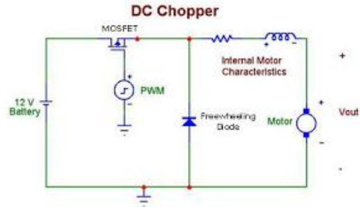
Gambar 2. Rangkaian aplikasi DC chopper
