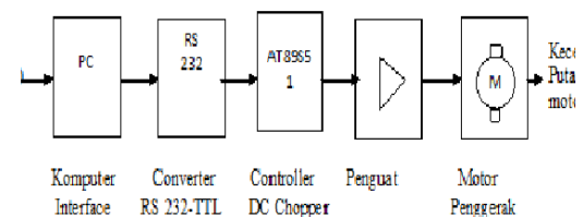
Gambar 3. Diagram blok sistem kerja pengaturan kecepatan Motor DC shunt
