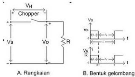
Gambar 1. Rangkaian pengelola DC-DC
