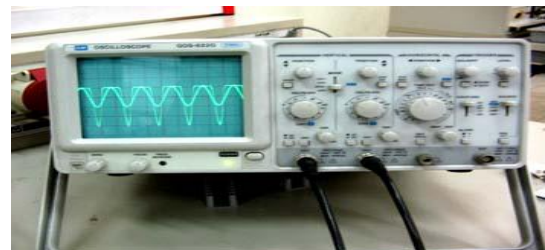
Gambar 4. Mengatur Garis Acuan Pada Osiloskop
