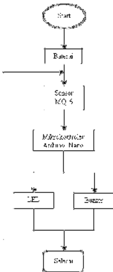
Gambar 5. Flowchart Sistem Kerja Alat
