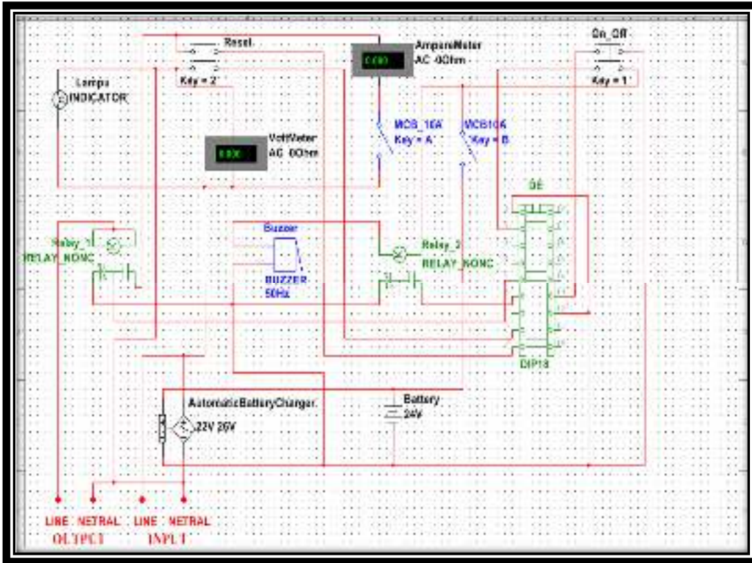
Gambar 4. Rangkaian Sistem Proteksi Menggunakan Modul Deep Sea 3110
