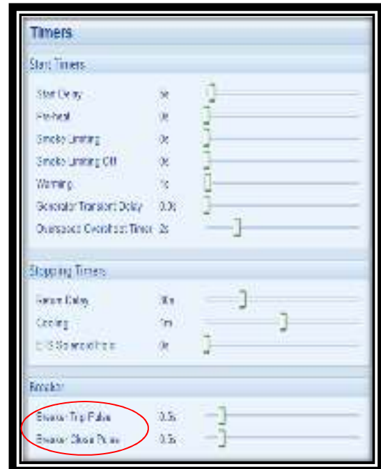
Gambar 7. Pengontrolan Timers pada Modul Deep Sea Elektronik 3110
