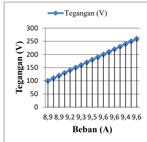
Gambar 5. Grafik Tegangan (V) VS Beban (A)
