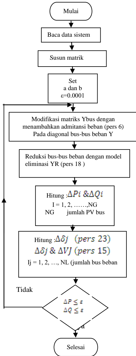
Gambar 2. Diagram Alir Modelisasi Eliminasi bus-bus beban
