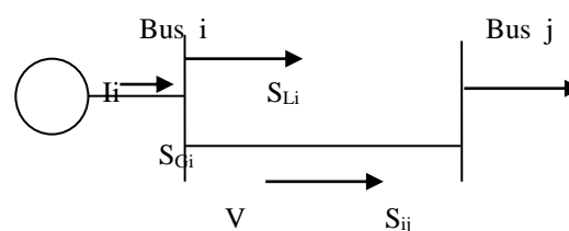
Gambar 1. Parameter Bus I dalam aliran beban
