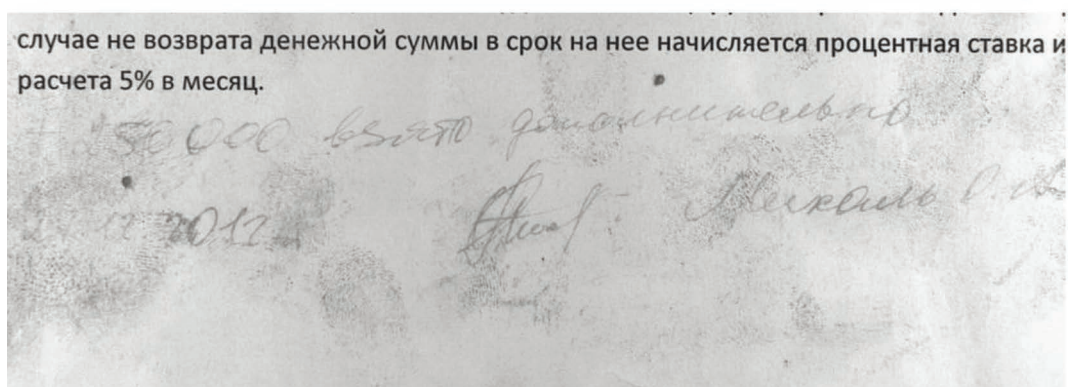
Рис. 15. Результат применения метода обработки парами кристаллического йода (внизу) исследованного документа (вверху) Fig. 15. A questioned document before (top) and after iodine fuming (bottom)
