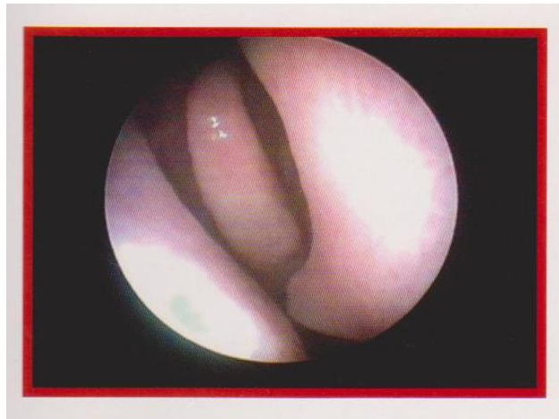
FIG. 8 : SEPTAL DEVIATION
