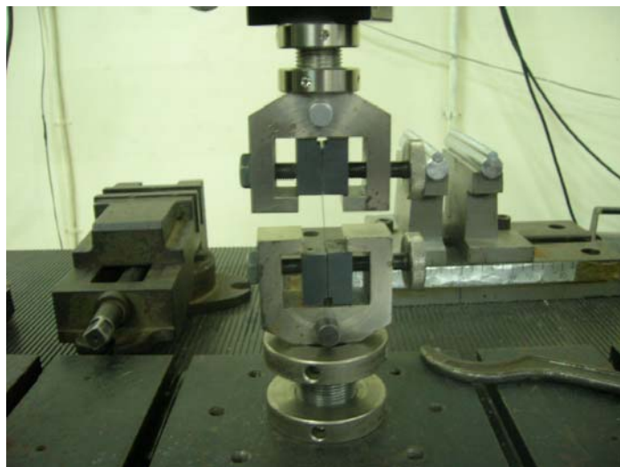
TENSILE TESTING
