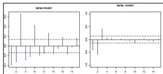
Gambar 1. Plot ACF dan PACF Data Simulasi
