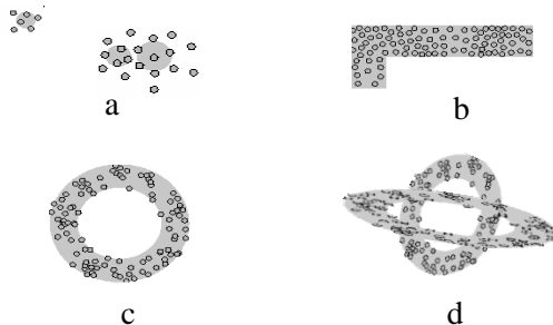
Gambar 2.1. Cluster dengan bentuk dan dimensi yang berbeda dalam \mathcal{R}^2 .
