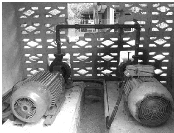
Figura 1. Bombas del sistema de bombeo.
