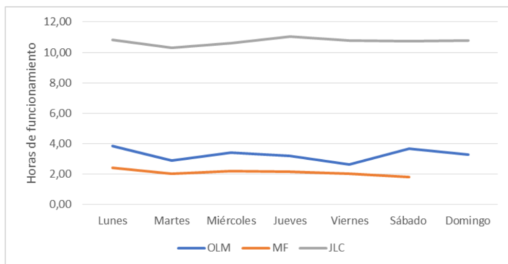
Figura 4. Tiempo de encendida la bomba en las tres sedes.
