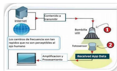
Figura 3. Transmisión de la señal LI-FI.
