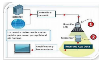
Figura 2. Funcionamiento del LI-FI
