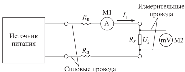
Рис. 4. Четырехпроводная схема измерения малых сопротивлений
