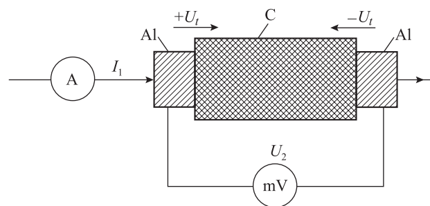
Рис. 6. Компенсация термоЭДС при измерении двумя токовыми электродами
