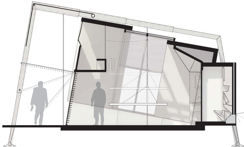
Section D-D
