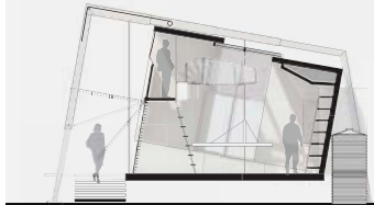
Section E-E Scale: 1/8" = 1'-0"
