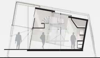
Section C-C Scale: 1/8" = 1'-0"
