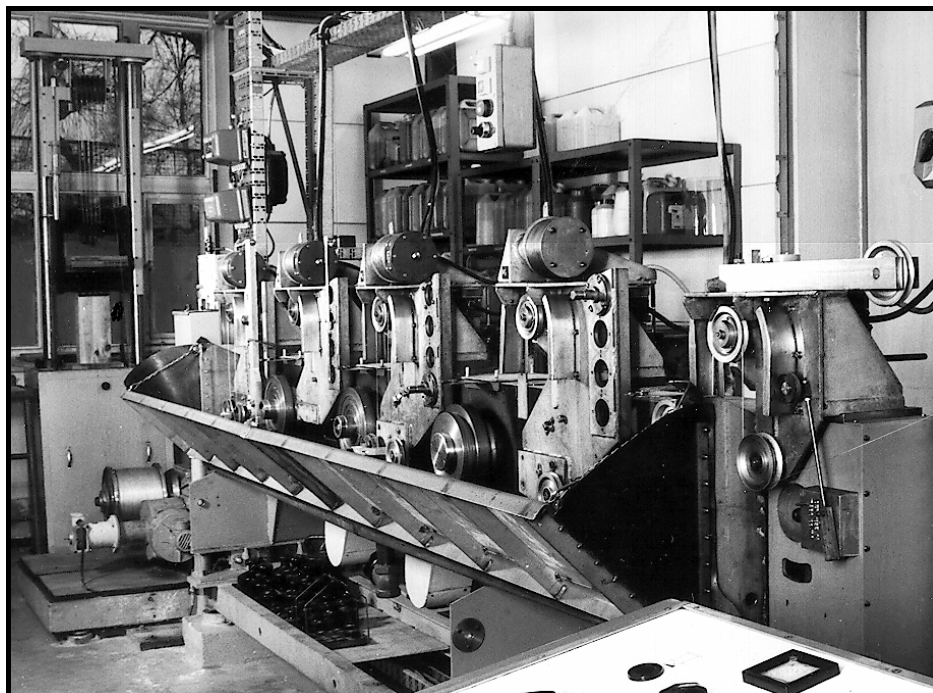
Bild 3.1.1-6: Labor-Feindrahtziehmaschine
