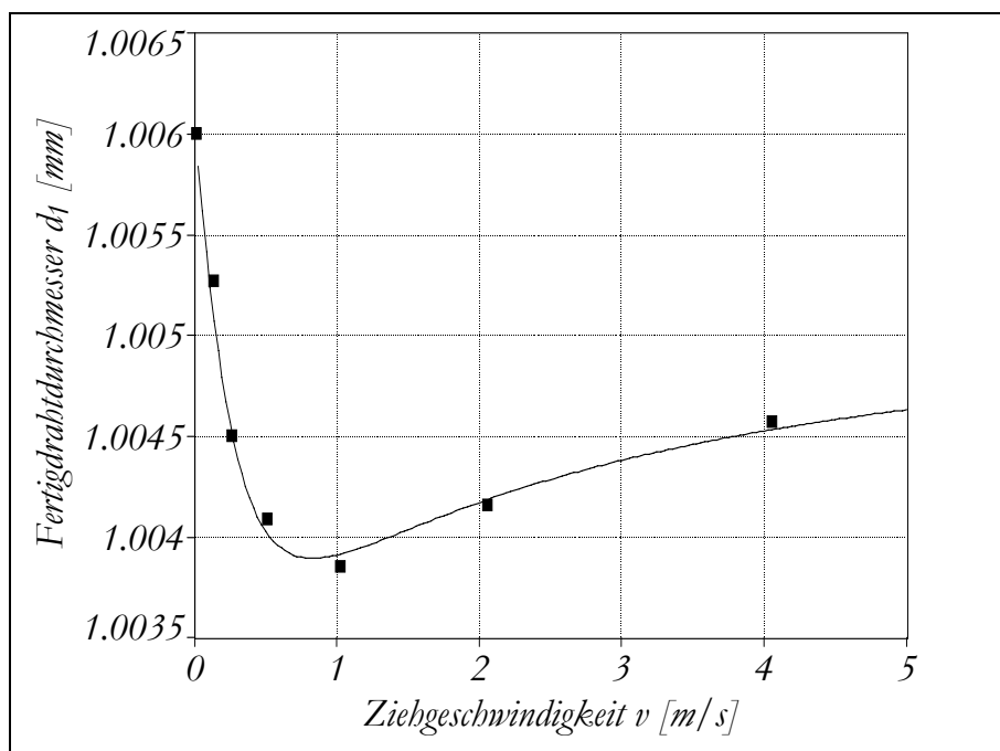
Bild 3.1.3-1: Fertigdrahtdurchmesseränderung (Plan 145, Versuch 1)
