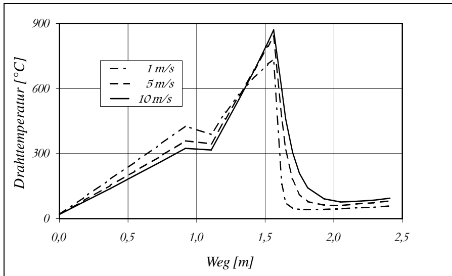
Bild 3.2-3.1: Temperatur-Weg-Abhängigkeit beim Durchlauf-Widerstandsglügen
