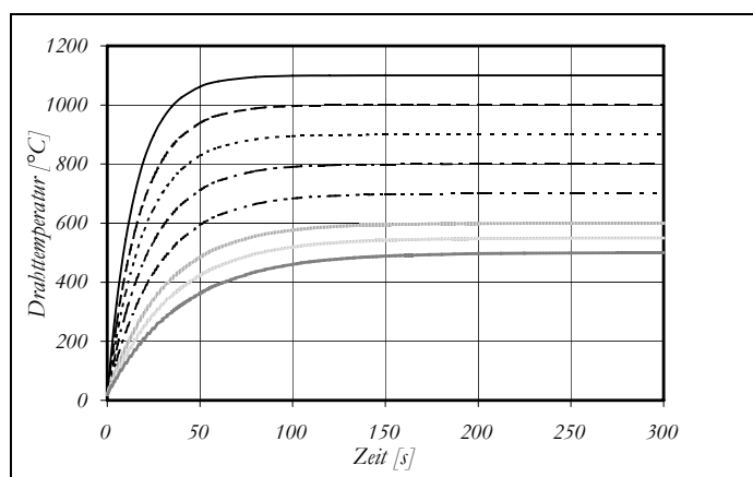
Bild 3.3-1: Drahterwärmung im Laborofen
