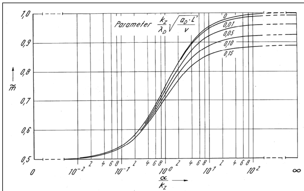
Bild 3.1.1-3: Mittlerer Wärmeverteilungskoeffizient bei Randbedingungen 2. Art
