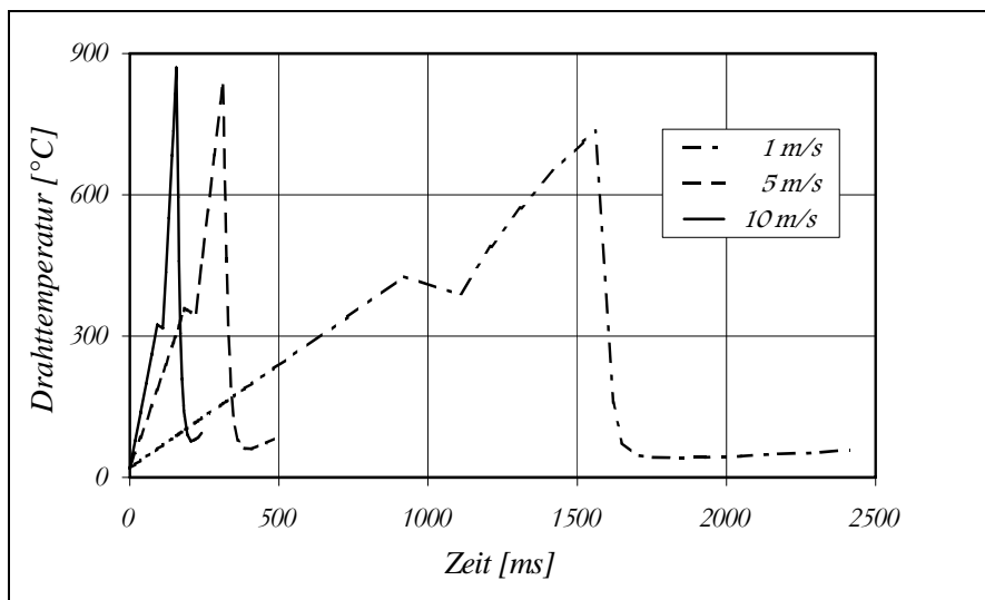
Bild 3.2-3.2: Temperatur-Zeit-Abhängigkeit beim Durchlauf-Widerstandsglügen
