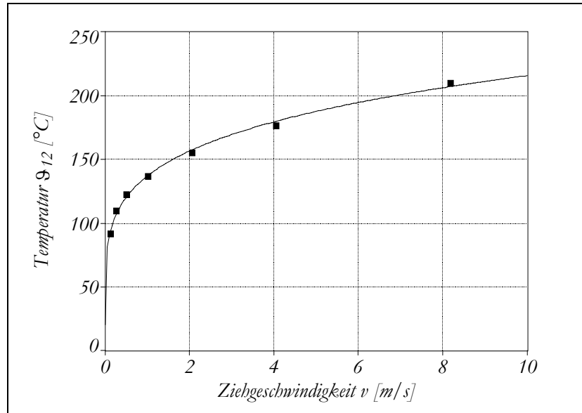
Bild 3.1.3-2: Ziehdüsentemperatur am Ziehholinnenrand
