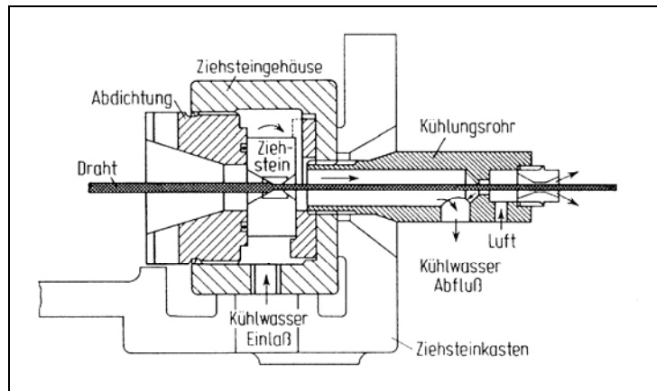
Bild 3.1.2-1: Kühlrohr-Wasserkühlung [NAK 76]
