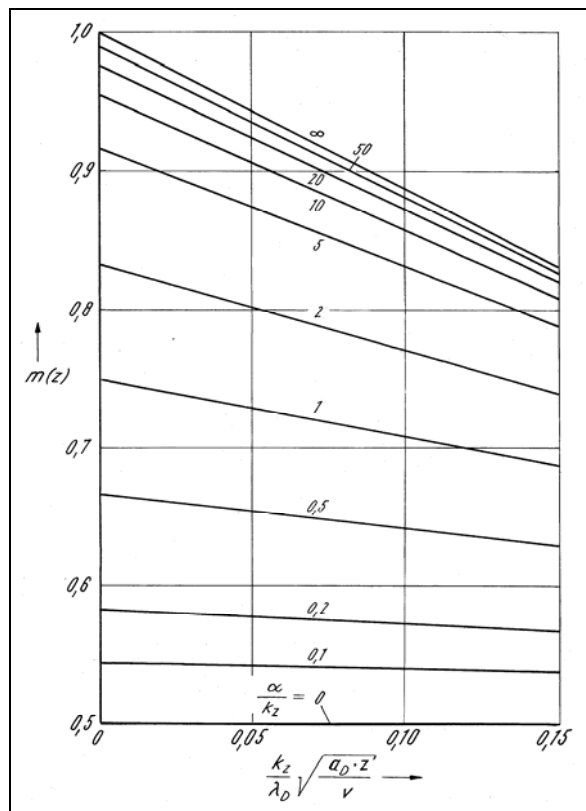
Bild 3.1.1-1: Wärmeverteilungsbeiwert bei Randbedingung 2. Art
