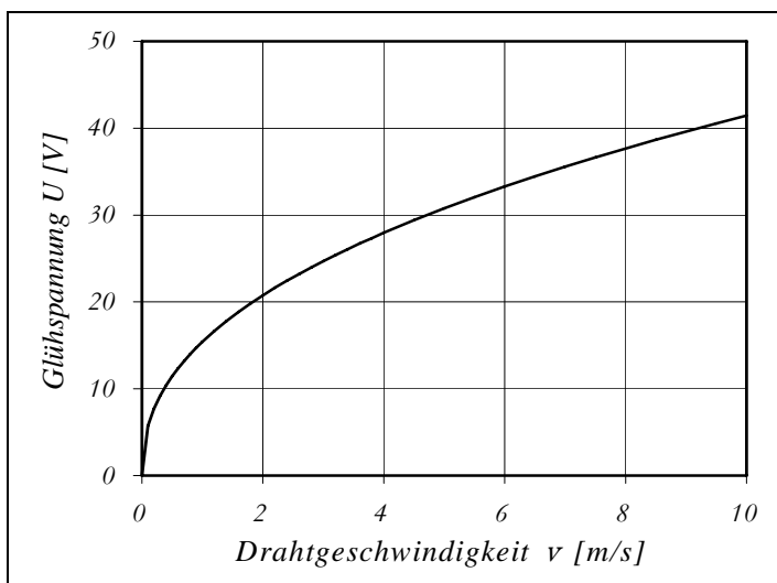
Bild 3.2-2: Glühspannungskurve für CuZn36-Draht
