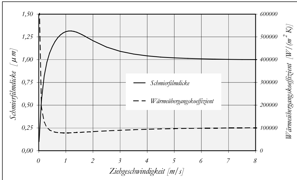
Bild 3.1.3-3: Schmierfilmdicke und Wärmeübergangskoeffizient
