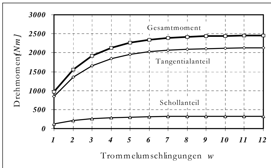
Bild A3.1.2-3: Anteile am Ziehtrommel-Lastdrehmoment
