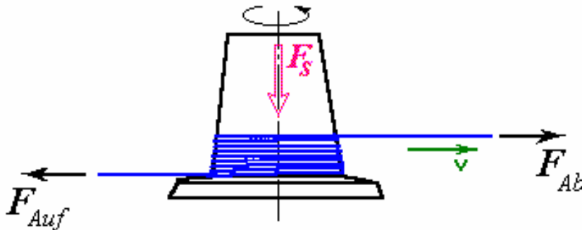
Bild A3.1.2-1: Kräfte an der Ziehtrommel
