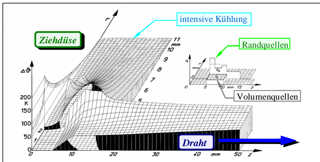
Bild 3.1.1-14: Temperaturfeld „Draht-Ziehdiüse“ mit idealisiert ortsabhängigem Schubspannungsverlauf
