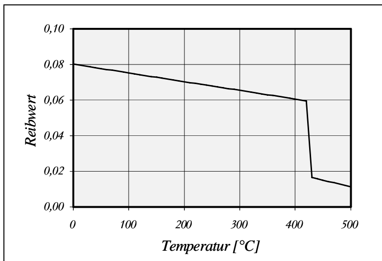
Bild 3.1.1-16: Reibwert-Temperaturabhängigkeit
