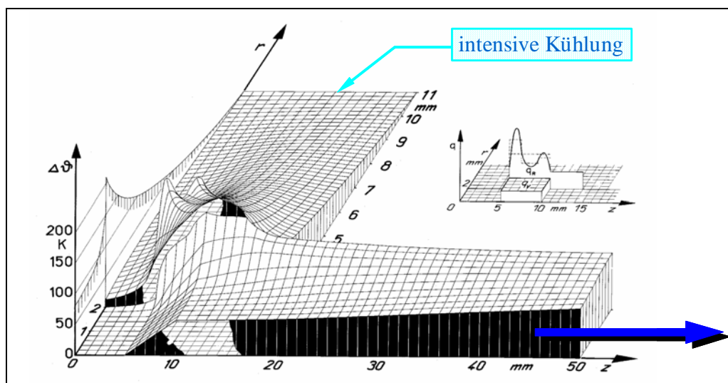
Bild 3.1.1-15: Temperaturfeld „Draht-Ziehdiüse“ mit real ortsabhängigem Schubspannungsverlauf
