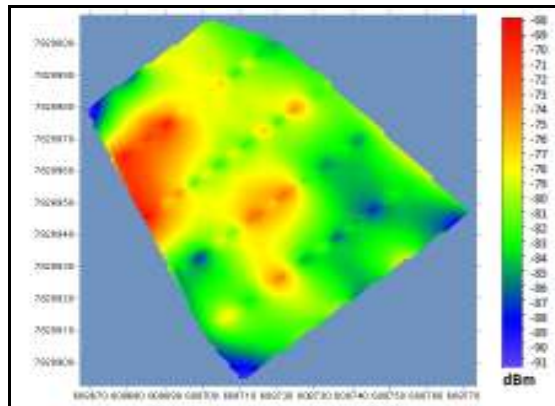
FIGURA 8. Mapa de zoneamento do sinal Wi-Fi correspondente ao MAC 002369B3D201.
