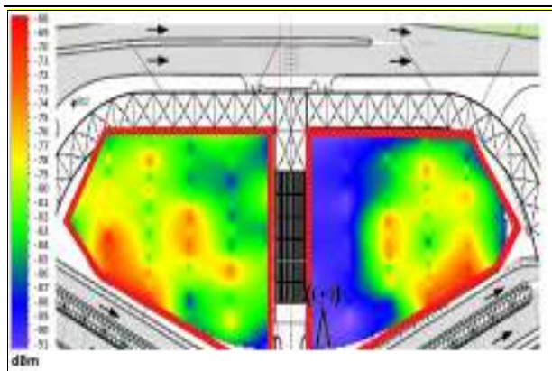
FIGURA 9. Planta baixa com os mapas de zoneamento de intensidade do sinal indicando a localização das antenas painéis na torre frontal (ícone).
