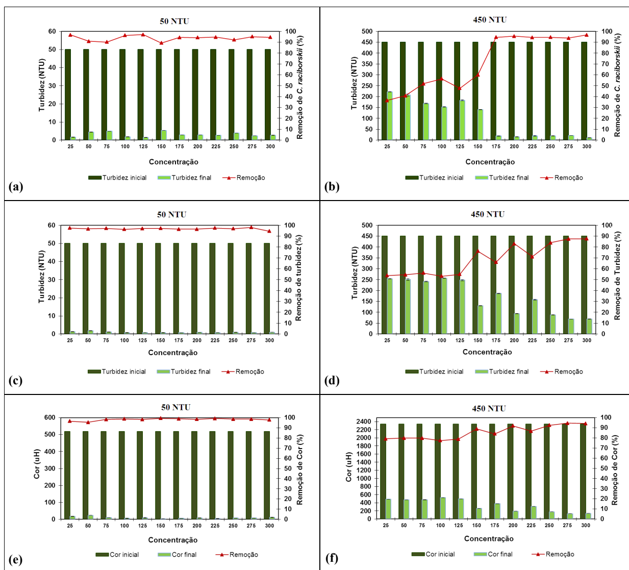
Figura 3 – Porcentagem de remoção para os diferentes valores de turbidez inicial: remoção de C. raciborskii (a) 50NTU, (b) 450 NTU; remoção de turbidez (c) 50NTU, (d) 450 NTU; remoção de cor aparente (e) 50NTU, (f) 450 NTU, usando o coagulante comercial Tanfloc SG.
