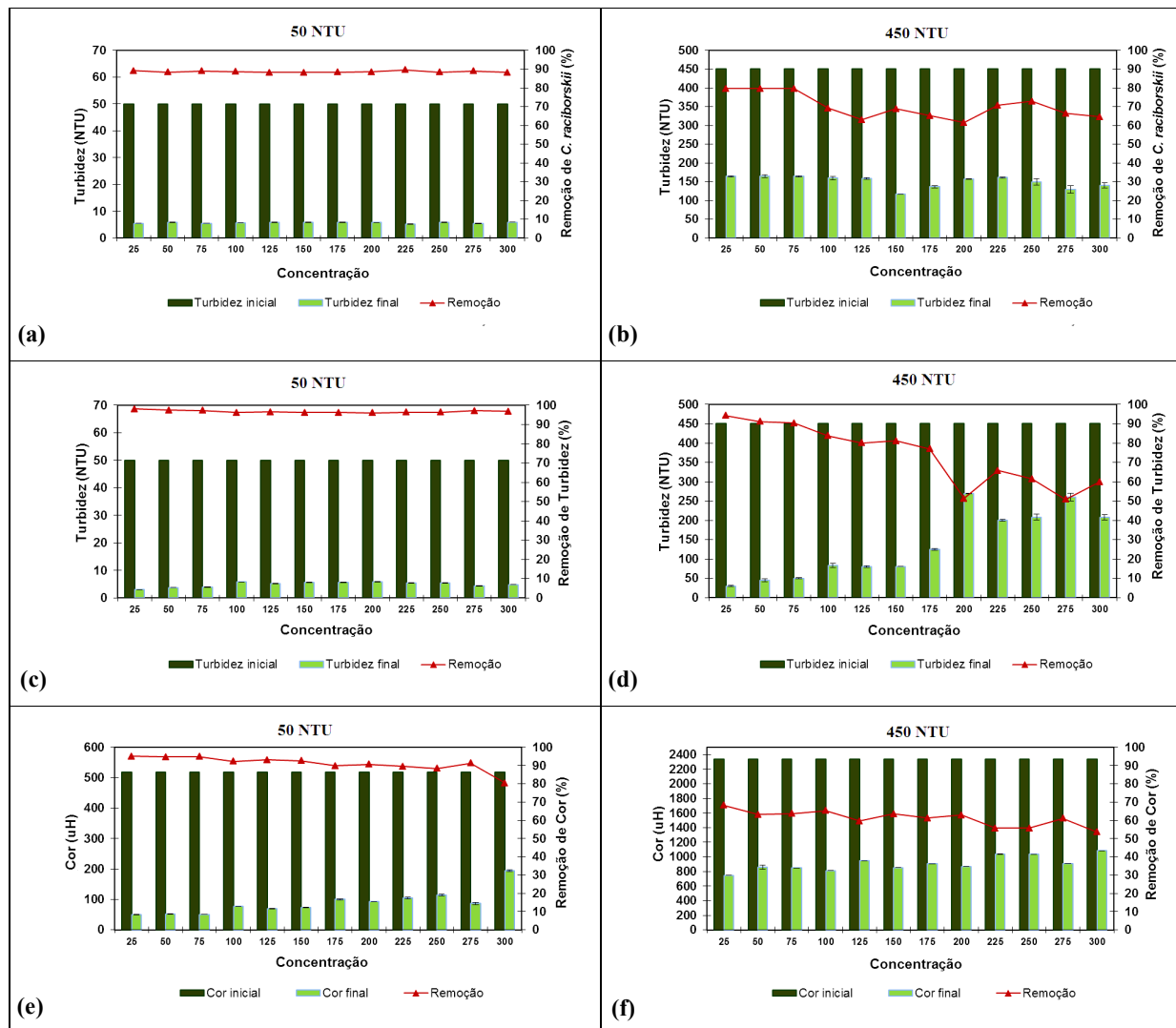
Figura 2 – Porcentagem de remoção para os diferentes valores de turbidez inicial: remoção de C. raciborskii (a) 50NTU, (b) 450 NTU; remoção de turbidez (c) 50NTU, (d) 450 NTU; remoção de cor aparente (e) 50NTU, (f) 450 NTU, usando a extração salina com NaCl (1M).
