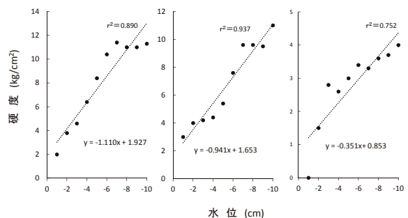
図10 潜砂実験における硬度と水位の関係
